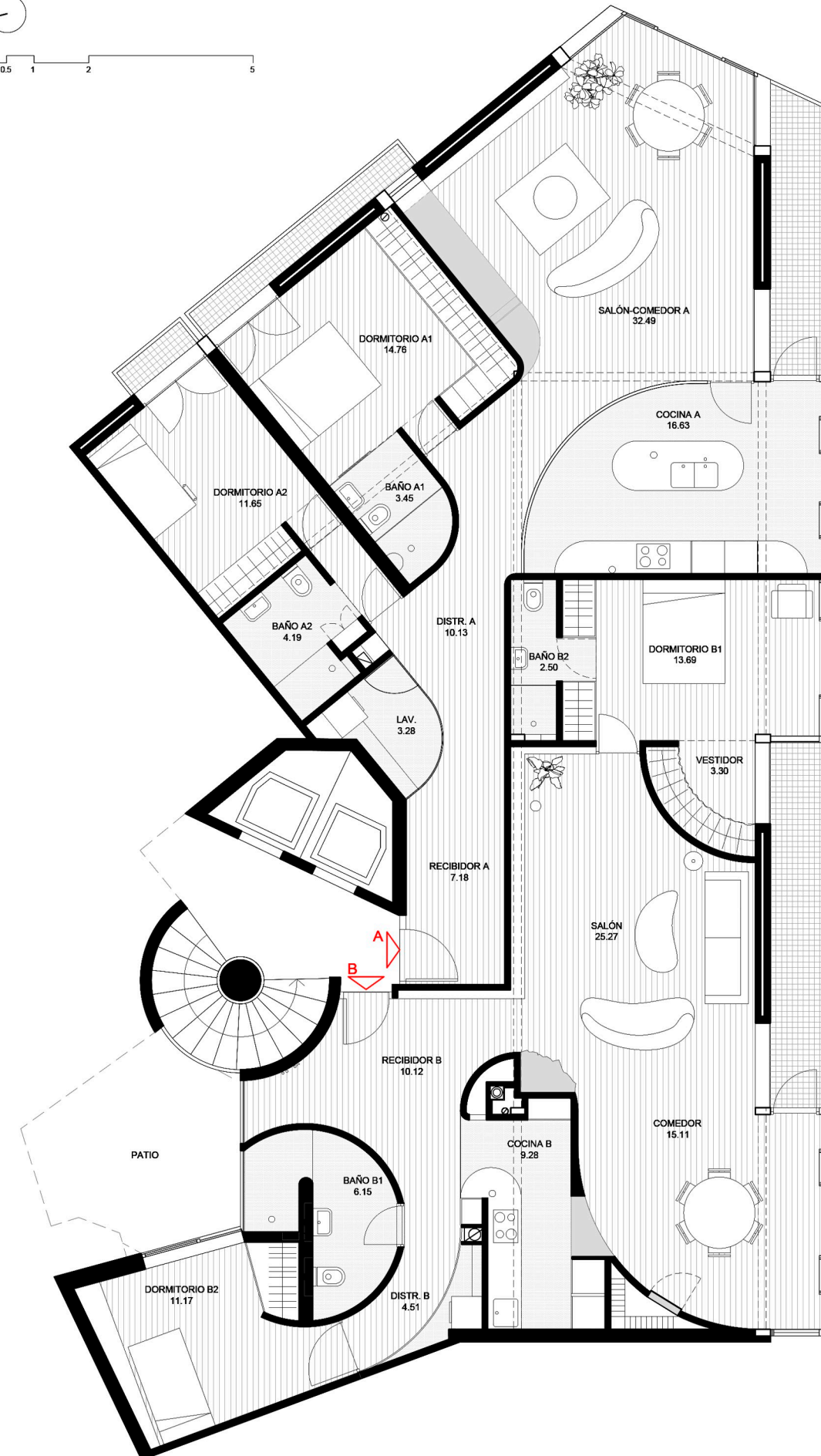
PLANTA. ESTADO REFORMADO
