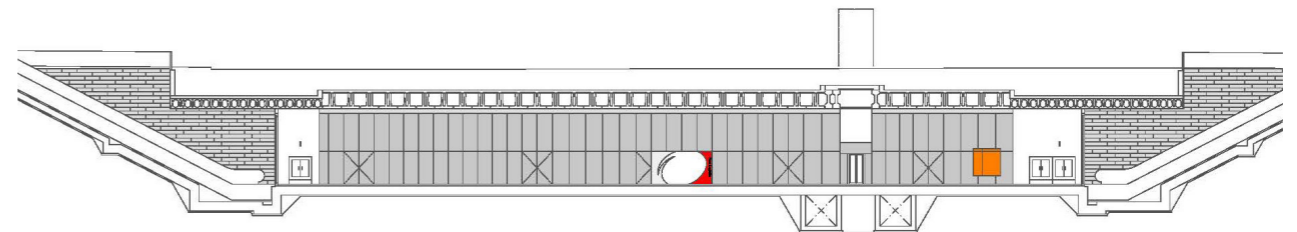
Sección B-B'
