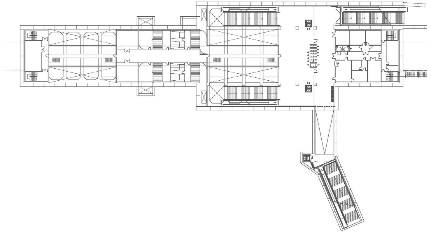
Planta vestíbulo
